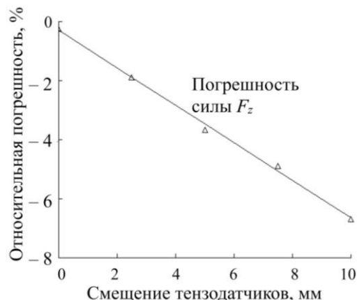
Рис. 5. Зависимость погрешности измерения силы от смещения парных тензодатчиков по вертикали вдоль оси z:
