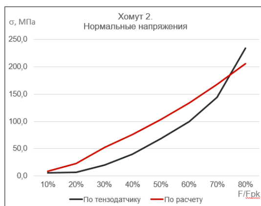
Рис. 11. Сравнение напряжений в хомутах № 2 (а) и № 3 (б) с результатами по расчетной модели
