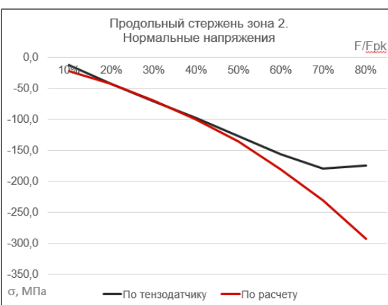
Рис. 12. Сравнение напряжений в продольных стержнях по тензодатчикам в зонах 1 (а) и 2 (б) с результатами по расчетной модели
