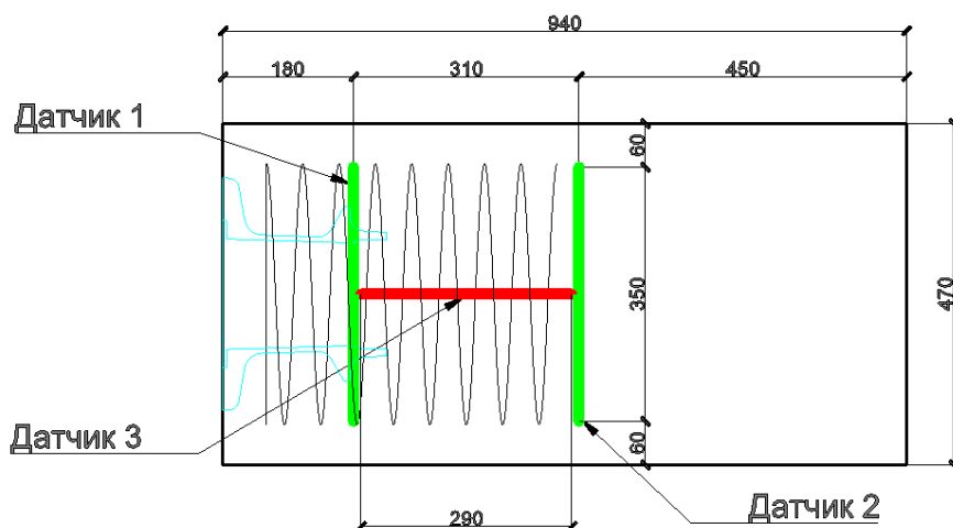
Рис. 5. Схема расположения баз индикаторов часового типа на грани призмы
