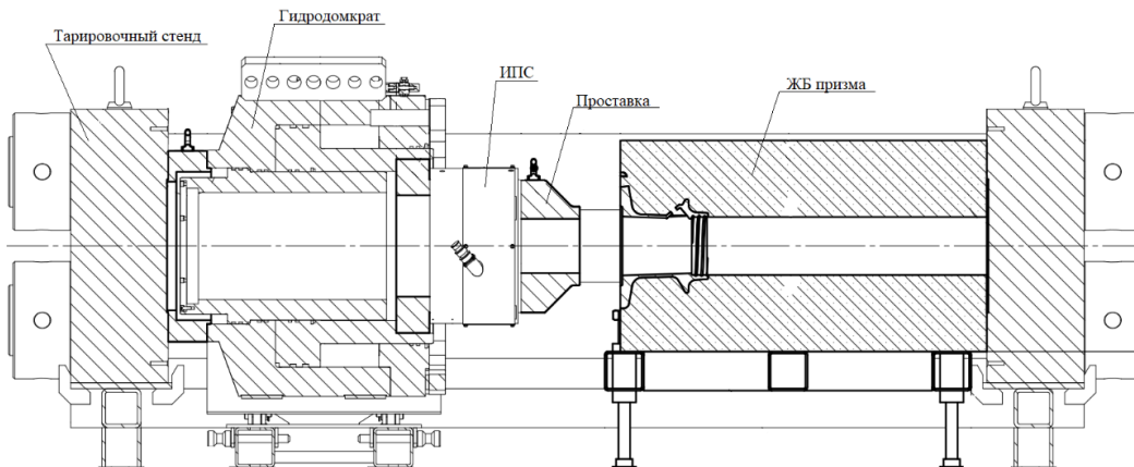
Рис. 7. Схема нагружения призмы в испытательном стенде
