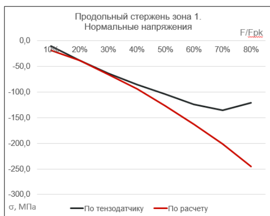
Рис. 12. Сравнение напряжений в продольных стержнях по тензодатчикам в зонах 1 (а) и 2 (б) с результатами по расчетной модели
