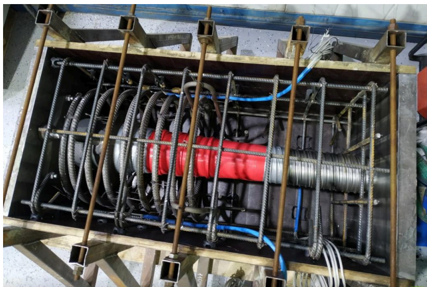
Рис. 2. Арматурный каркас и элементы СПН в опалубке
