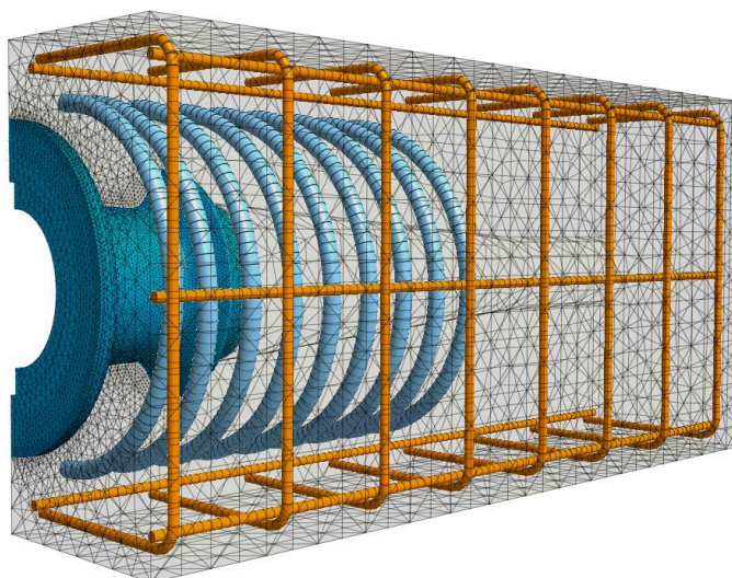
Рис. 9. Расчетная модель испытательной призмы в MIDAS FEA NX
