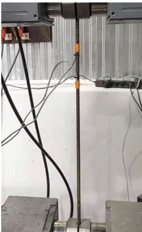
Рис. 3. Процесс испытания арматурного стержня (а) с наклеенным тензодатчиком (б)
