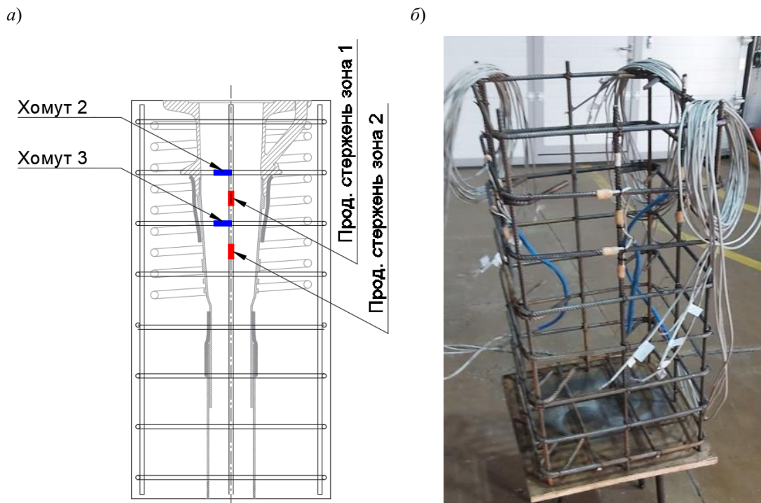
Рис. 4. Схема расположения тензодатчиков в арматурном каркасе призмы (а), а также фактически смонтированные на каркас тензодатчики (б)
