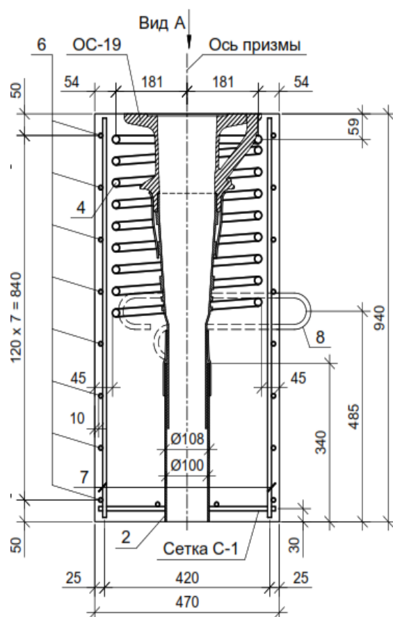
Рис. 1. Фрагмент рабочей документации на железобетонную призму
